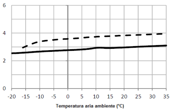
Consumo elettrico (kW)
